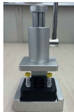
プレス機
